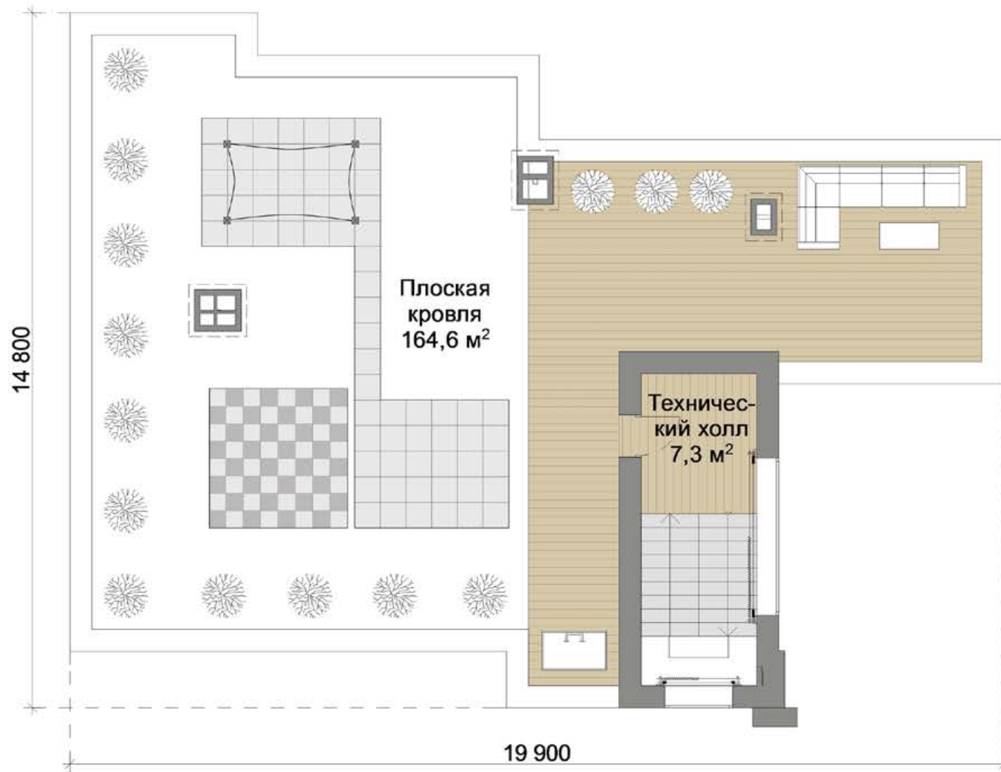
План 3-ого этажа Общая площадь: 171,9 м 2
